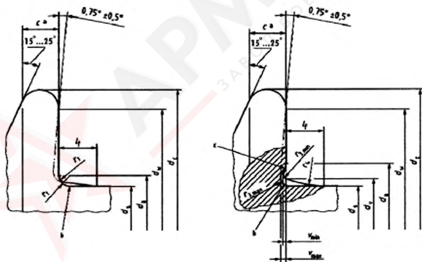
Рисунок 2 – Болт с шестигранной головкой с фланцем – уменьшенный стержень, тип R (по запросу)
