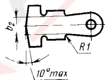
Развертка Рис 3 Остальное см рис 1
