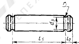
Тип 4 (под запорное кольцо)
